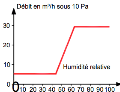
Entrées d'air hygroréglables
