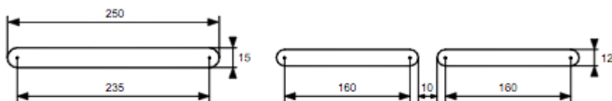
Exemples de fentes standards
